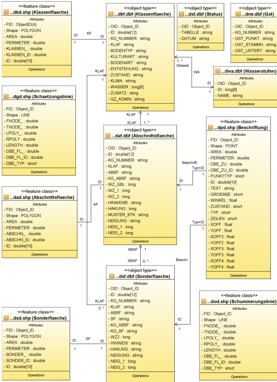
Abbildung 4: DBE-Datenmodell
